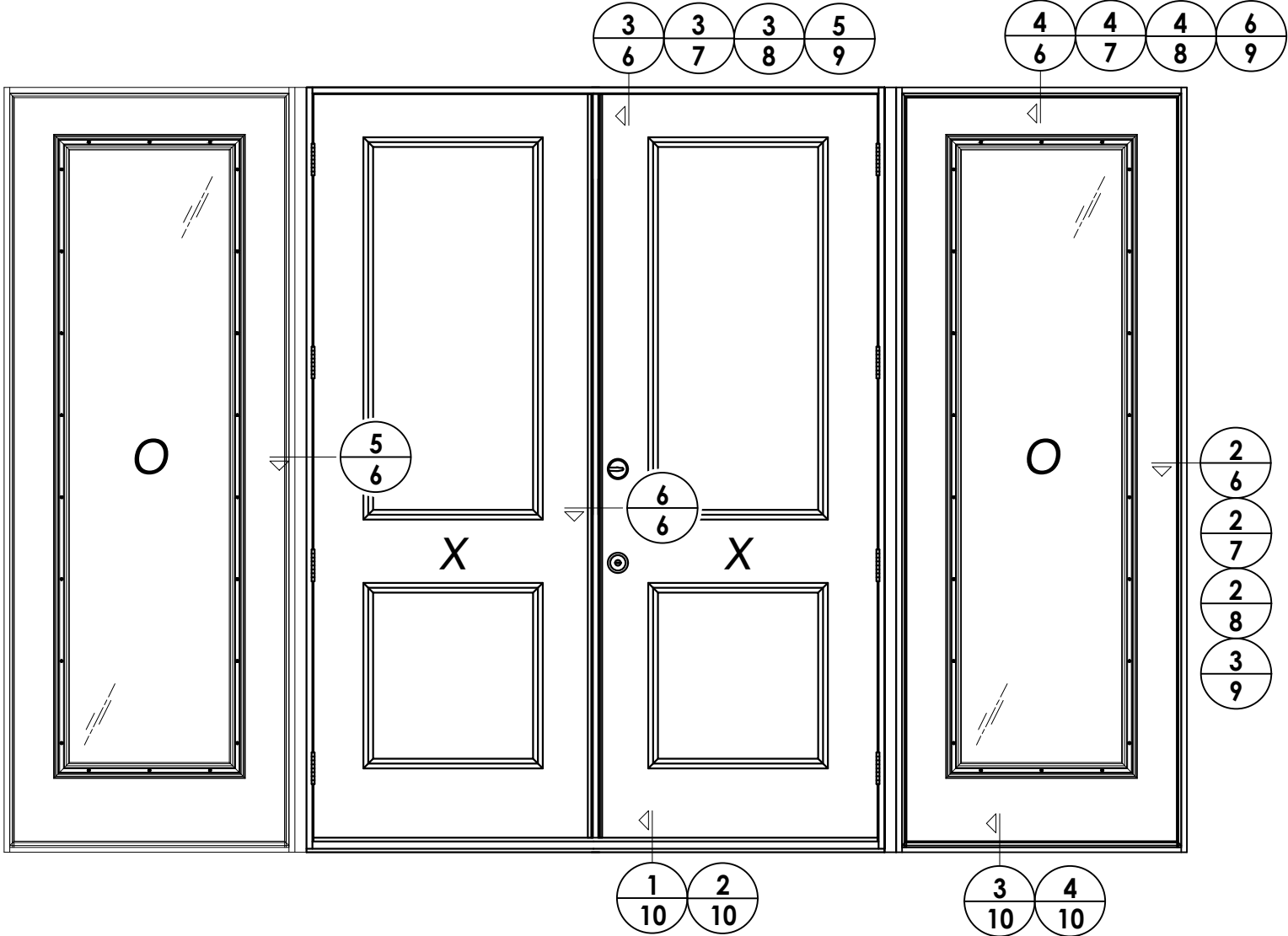
ELEVATION (OXXO)
